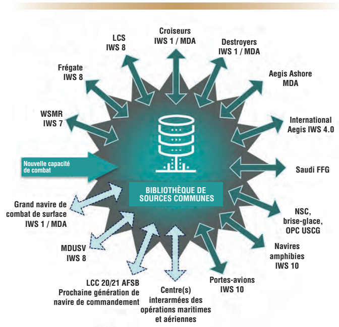
Figure 3. Navires équipés d'Aegis utilisant la référence logicielle Common Source Library.
