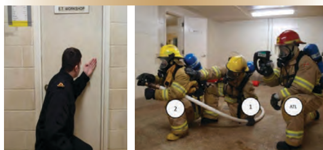
Figure 1. Intervention à deux niveaux de la MRC en cas d'incendie à bord d'un navire : Une vérification de la température à l'arrière de la porte par un membre de l'équipe d'intervention rapide, suivie d'une équipe d'attaque entièrement équipée, armée d'une caméra d'imagerie thermique.
