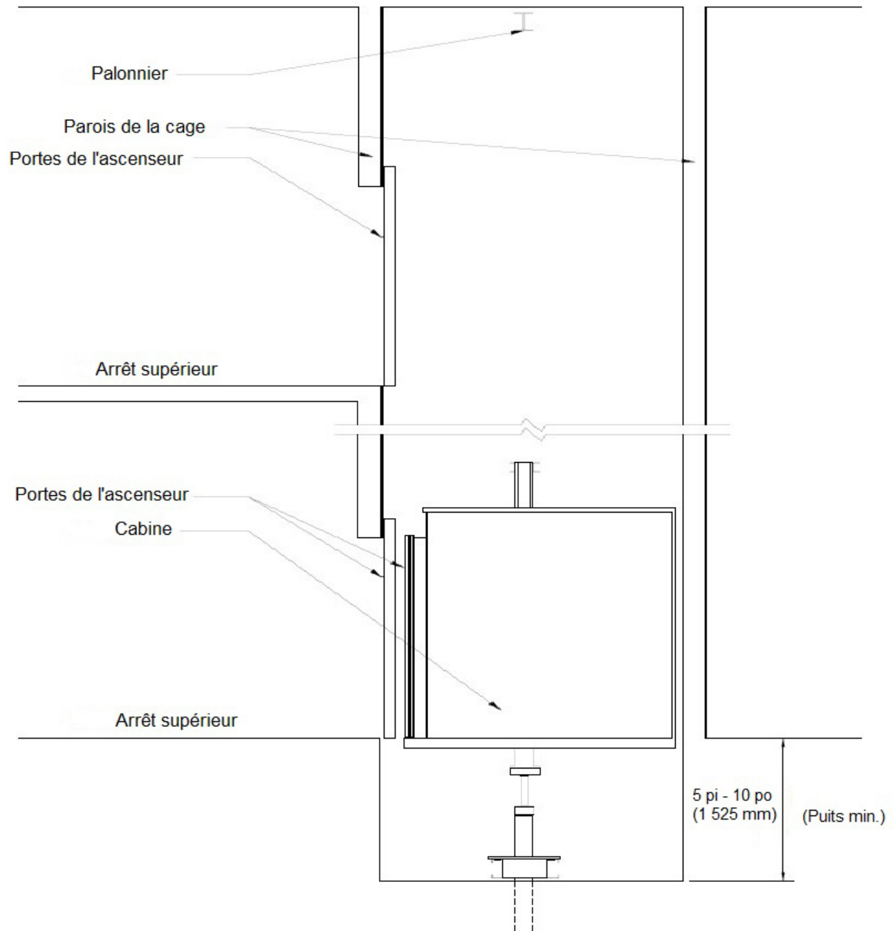
Figure 11 : Ascenseur hydraulique
