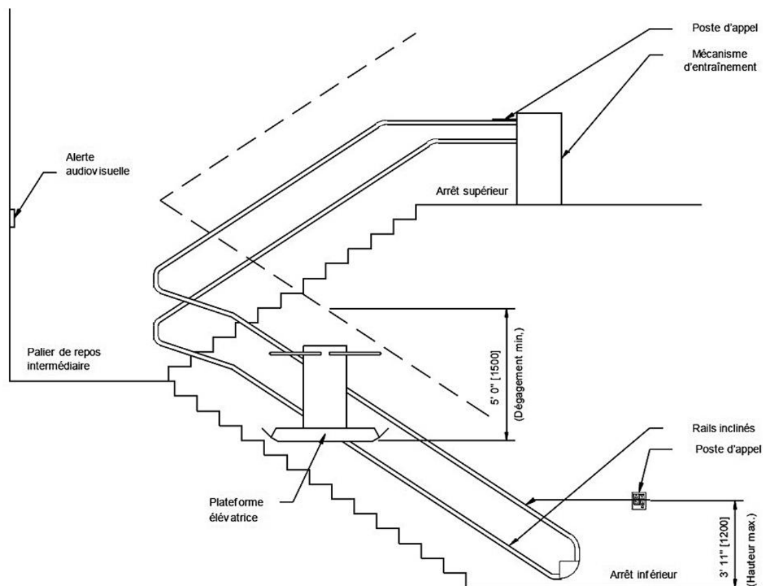
Figure 8 : Plateforme élévatrice inclinée
