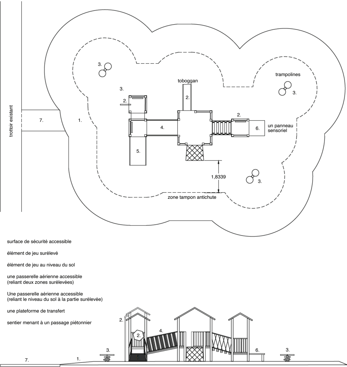
Figure 19 : Aire de jeu accessible - grande
