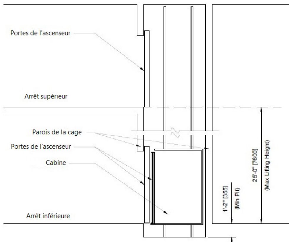
Figure 10 : Ascenseur à usage limité/utilisation limitée (ULUL)
