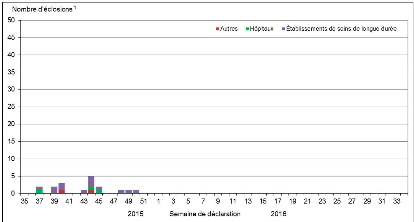
Figure 5 – Nombre total de nouvelles éclosions de la grippe confirmée en laboratoire par semaine, Canada, 2015-16
