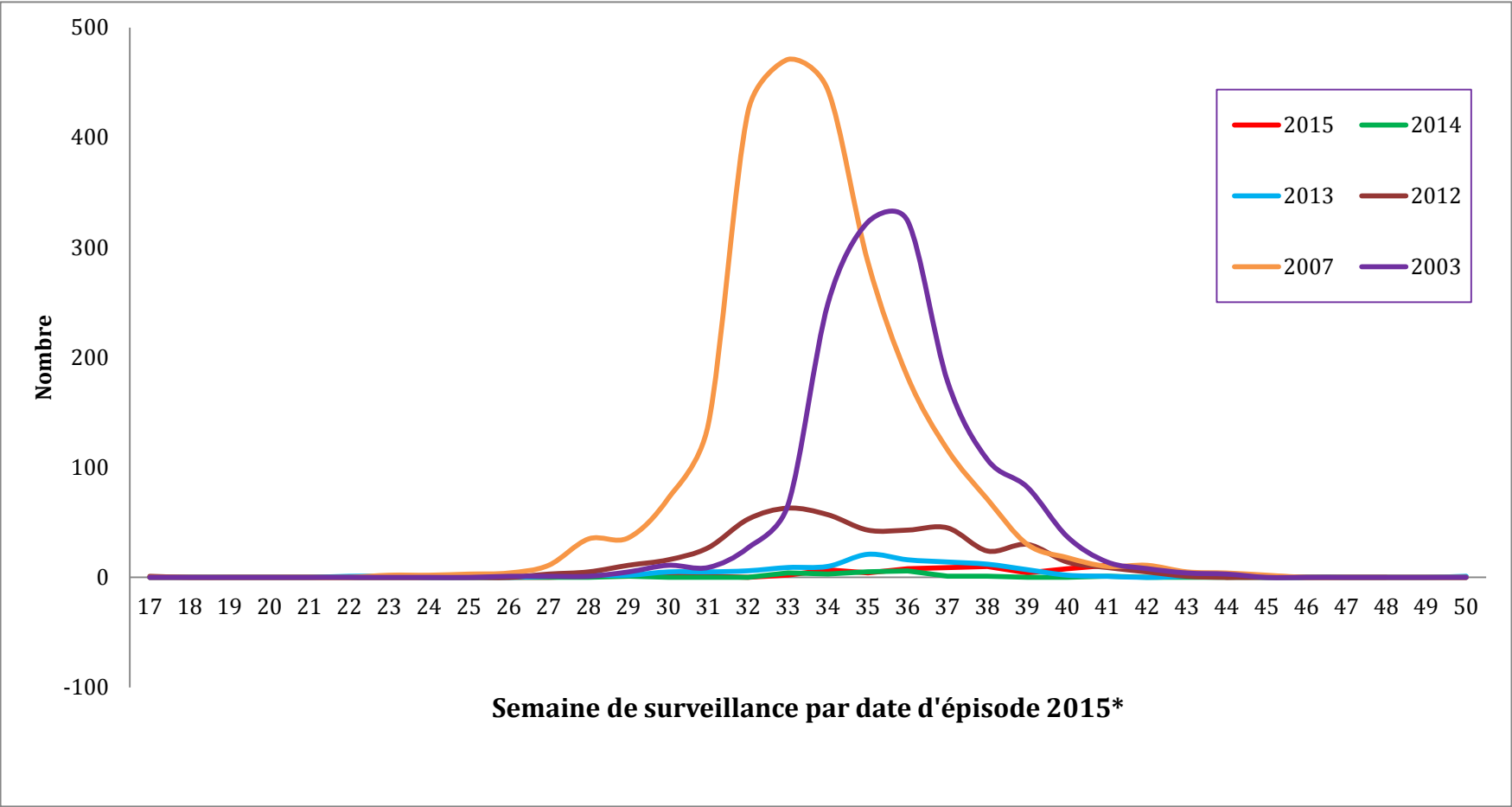
FIGURE 2 : Cas cliniques et infections asymptomatiques associés au virus du Nil occidental, par semaine de déclaration, au cours de certaines anné
