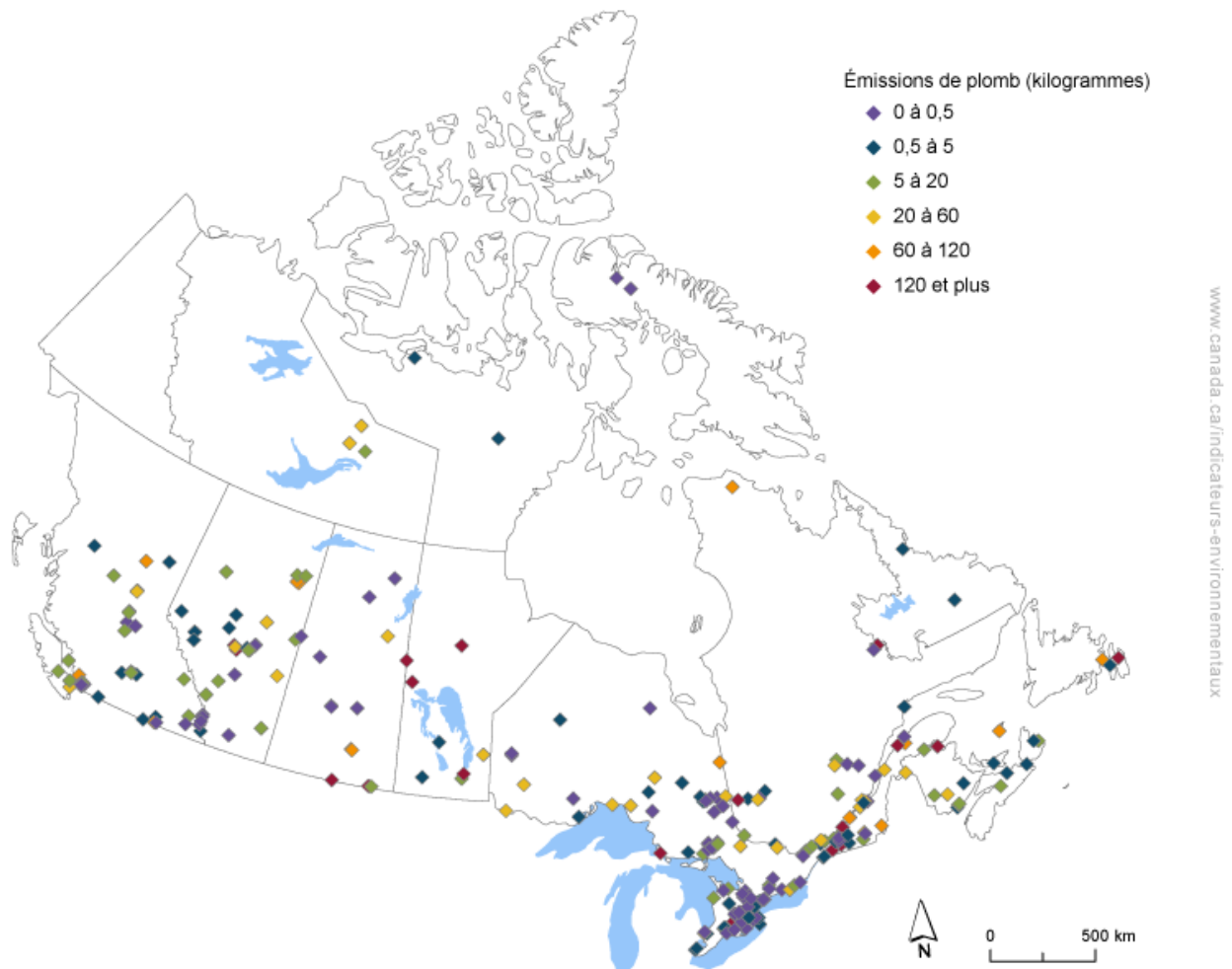
Figure 8. Émissions atmosphériques de plomb par installation, Canada, 2016
