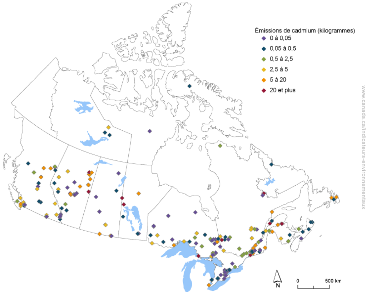
Figure 11. Émissions atmosphériques de cadmium par installation, Canada, 2016
