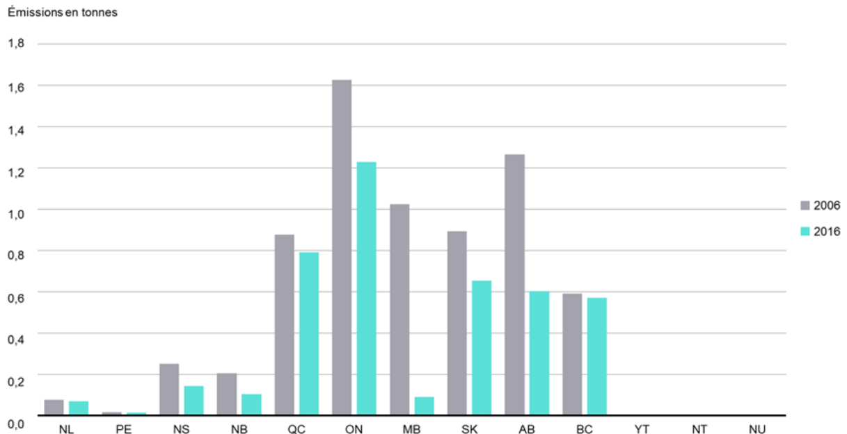
Figure 3. Émissions atmosphériques de mercure par province et territoire, Canada, 2006 et 2016
