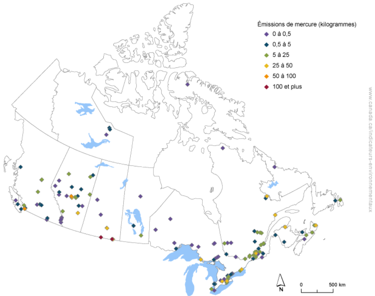
Figure 4. Émissions atmosphériques de mercure par installation, Canada, 2016
