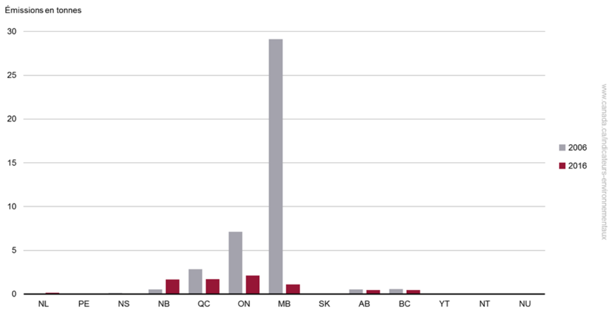
Figure 10. Émissions atmosphériques de cadmium par province et territoire, Canada, 2006 et 2016
