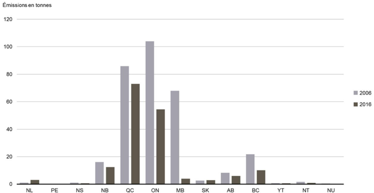
Figure 7. Émissions atmosphériques de plomb par province et territoire, Canada, 2006 et 2016
