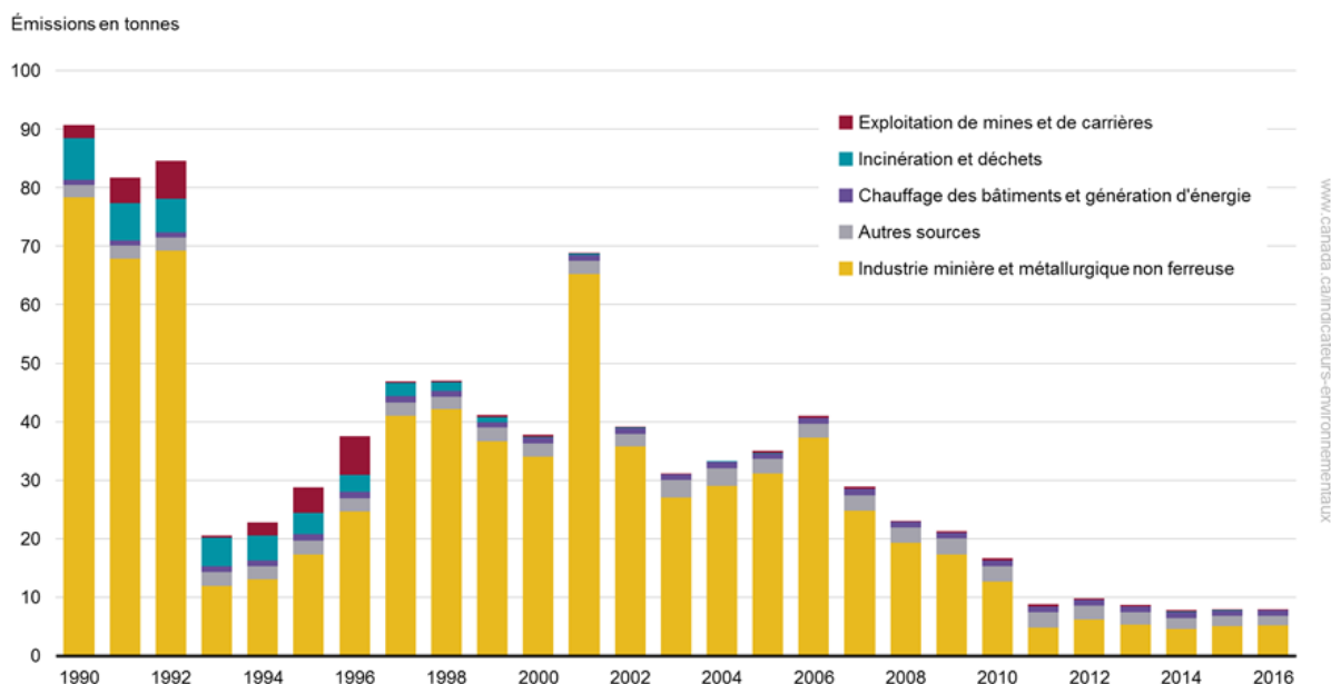
Figure 9. Émissions atmosphériques de cadmium par source, Canada, 1990 à 2016
