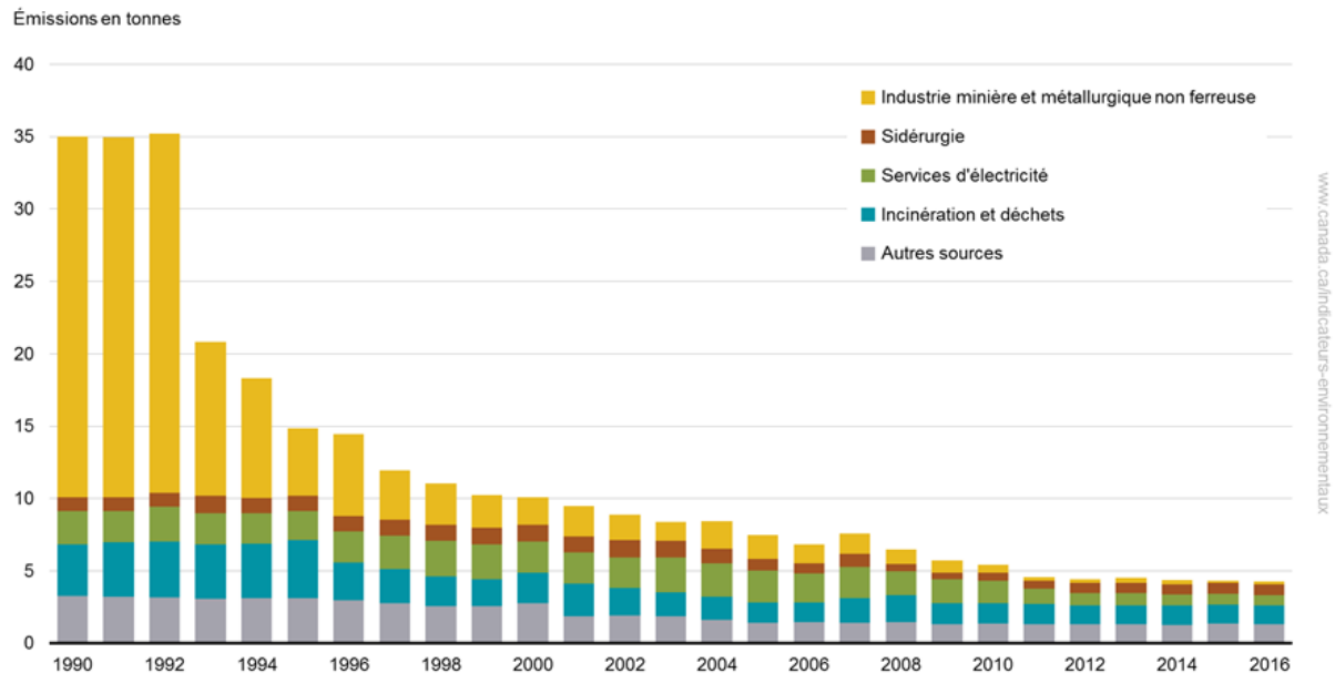
Figure 2. Émissions atmosphériques de mercure par source, Canada, 1990 à 2016
