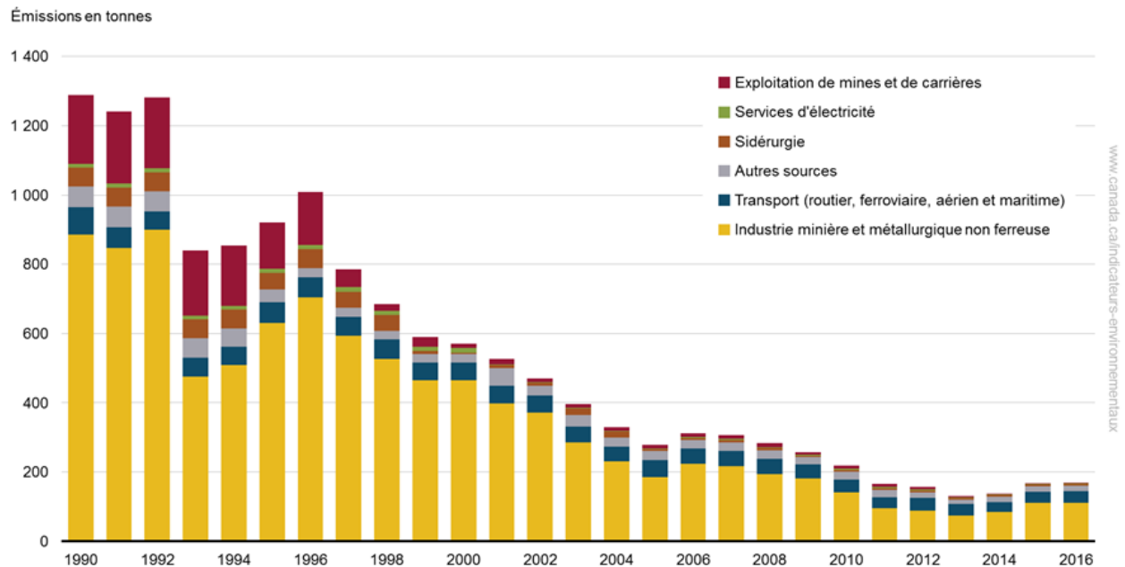
Figure 6. Émissions atmosphériques de plomb par source, Canada, 1990 à 2016
