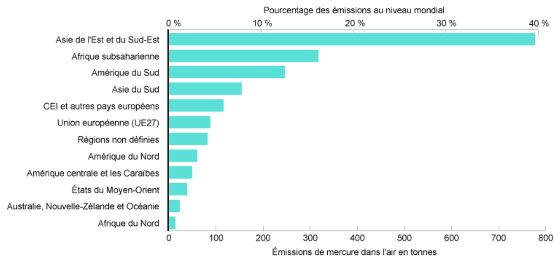
Figure 5. Émissions atmosphériques mondiales de mercure, 2010
