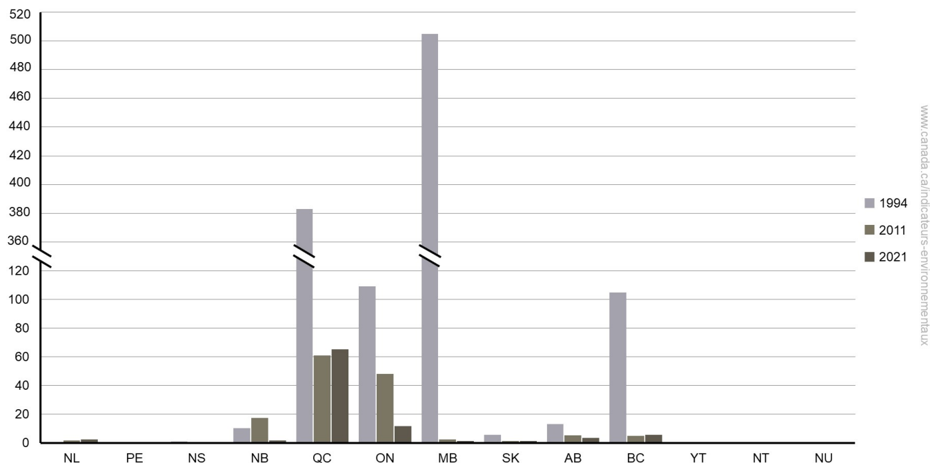
Figure 7. Émissions atmosphériques de plomb par province et territoire, Canada, 1994, 2011 et 2021 Émissions en tonnes
