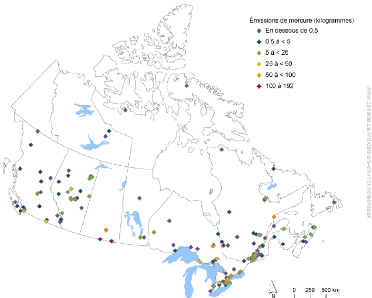
Figure 4. Émissions atmosphériques de mercure par installation, Canada, 2021
