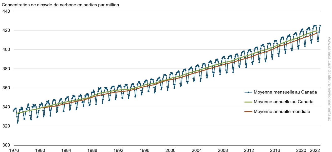
Figure 1. Concentration de dioxyde de carbone, Canada et à l'échelle mondiale, 1976 à 2022
