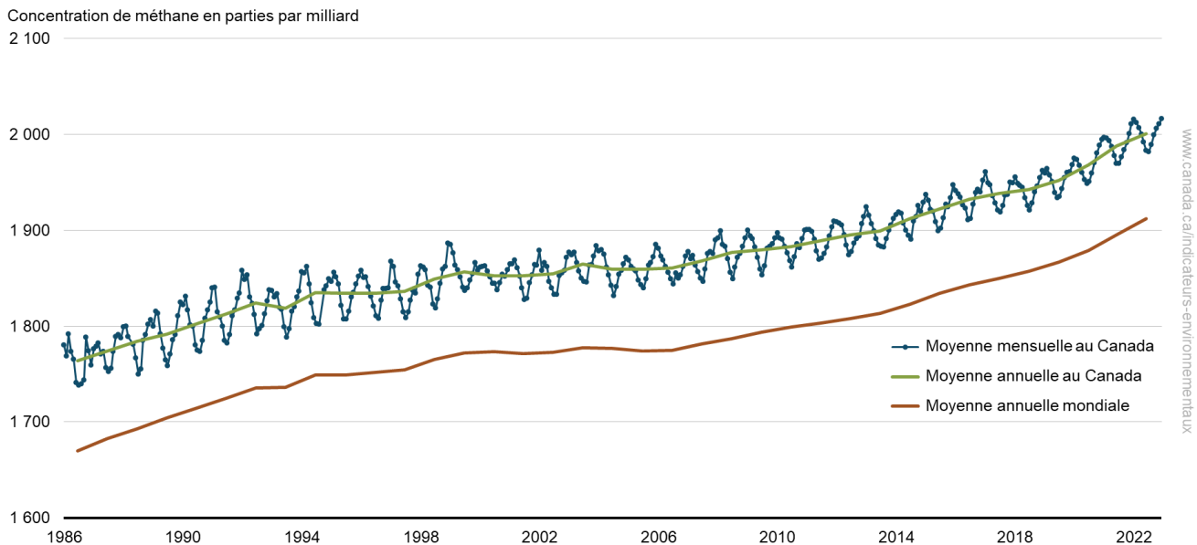
Figure 2. Concentration de méthane, Canada et à l'échelle mondiale, 1986 à 2022
