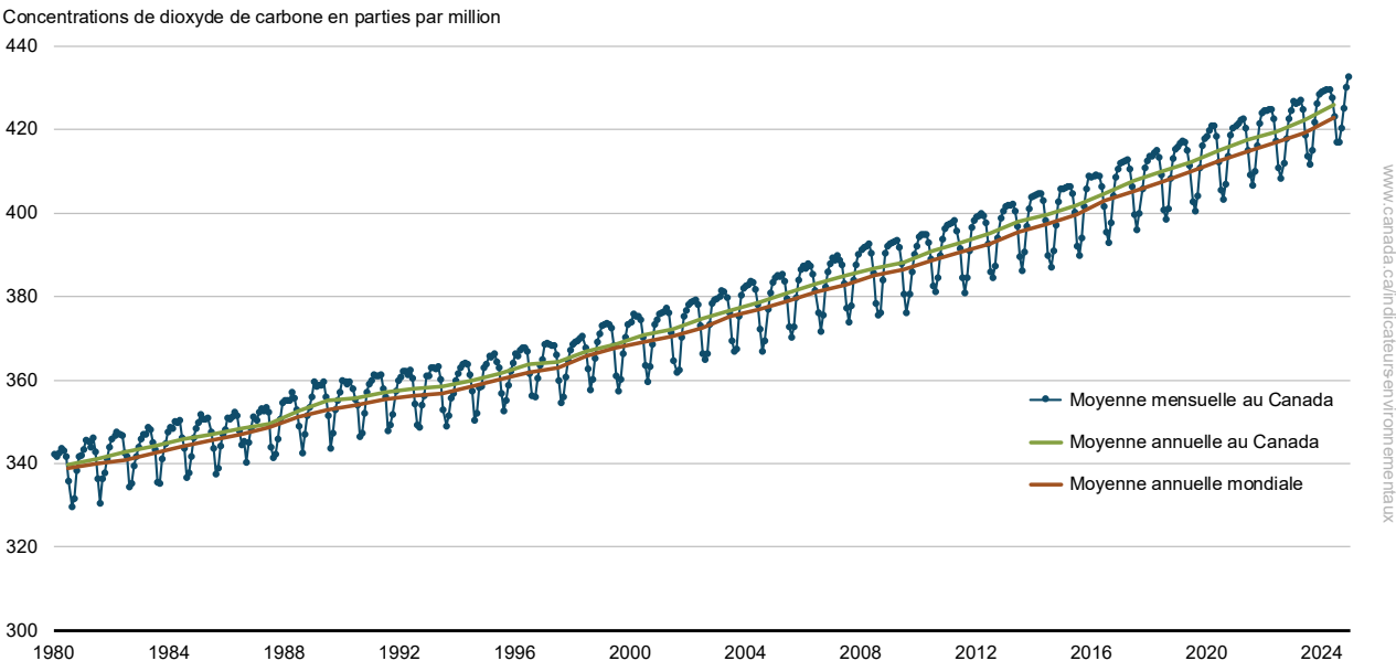
Figure 1. Concentrations de dioxyde de carbone, Canada et à l'échelle mondiale, 1980 à 2024
