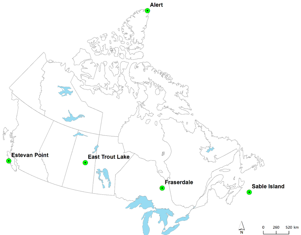
Figure 3. Stations de surveillance de concentrations de gaz à effet de serre au Canada, 2025
