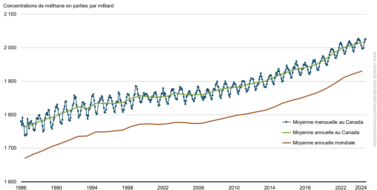
Figure 2. Concentrations de méthane, Canada et à l'échelle mondiale, 1986 à 2024
