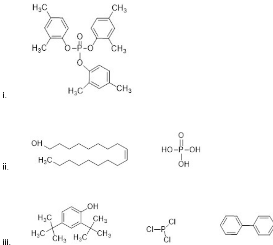
Figure 1. Structures chimiques des substances du groupe des acides phosphoriques et dérivés
