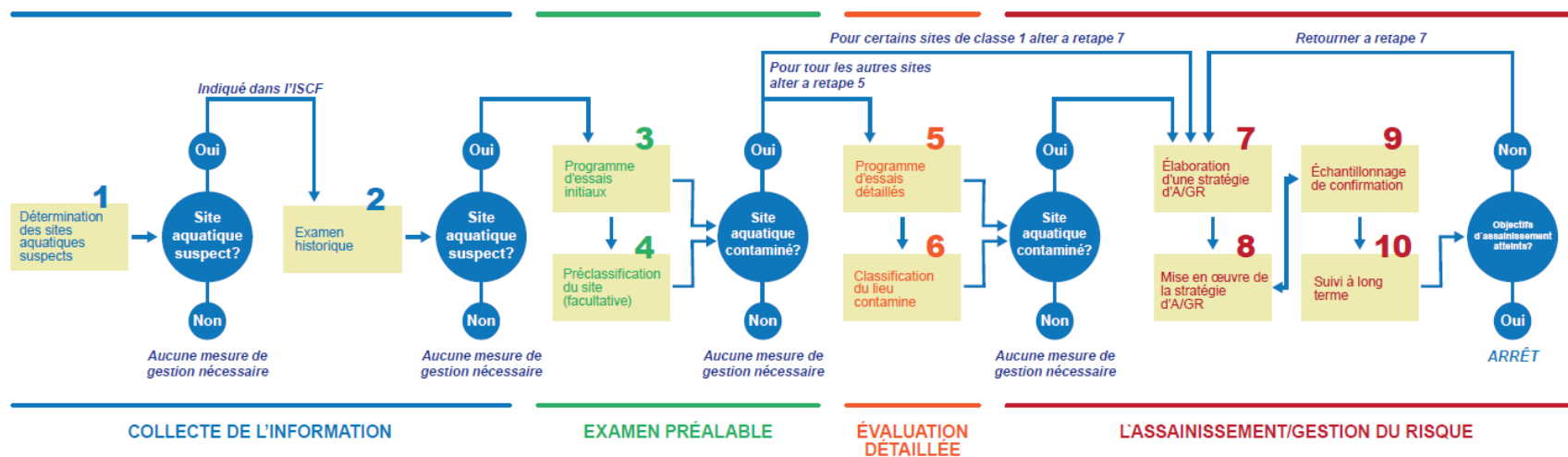
Figure 1 : Étapes de l'évaluation et de la gestion des sites aquatiques contaminés
