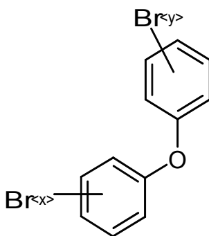
Figure 1. Structure de base des PBDE examinés dans la présente évaluation, où x + y = 4-10
