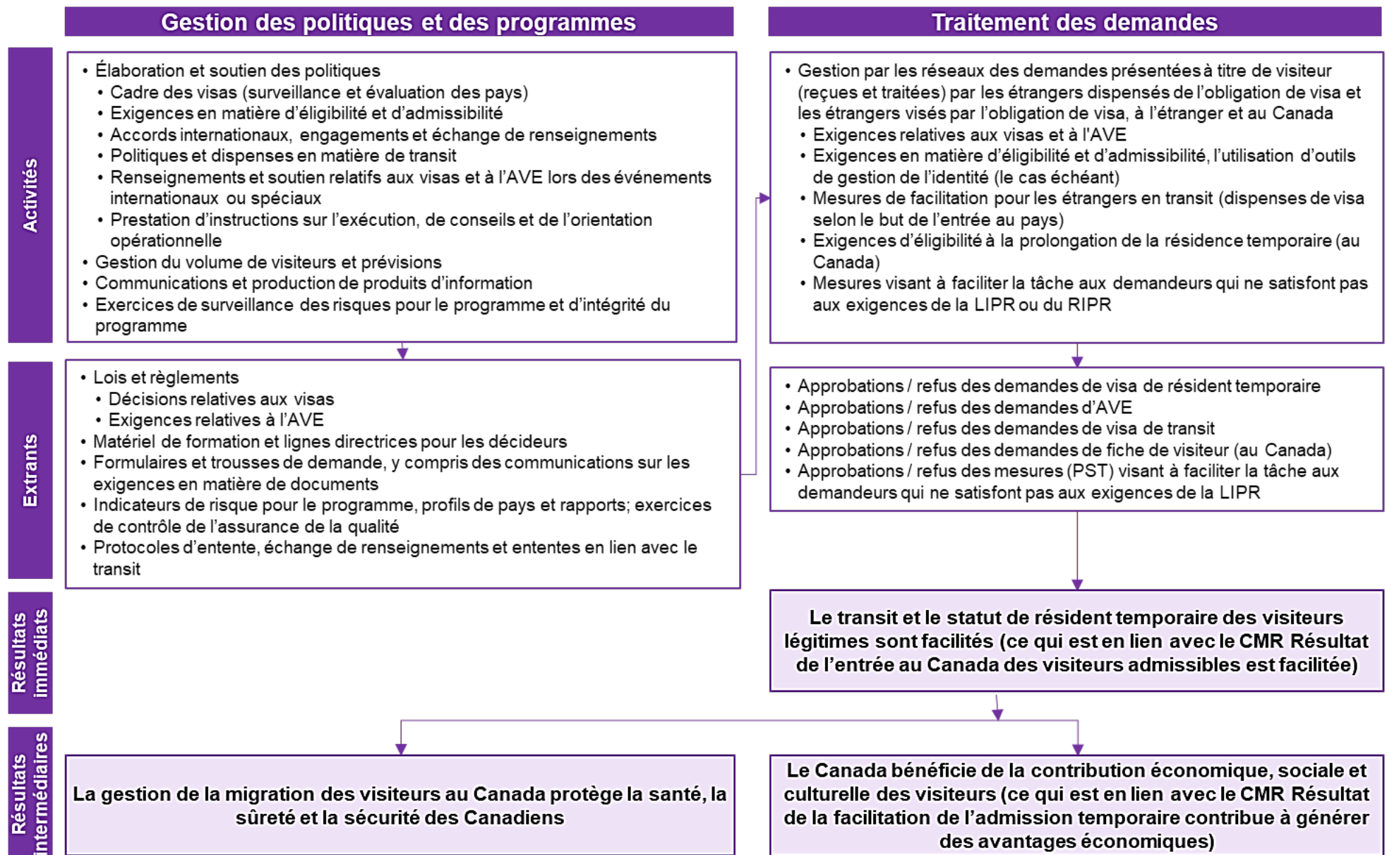
Figure 9 : Modèle logique
