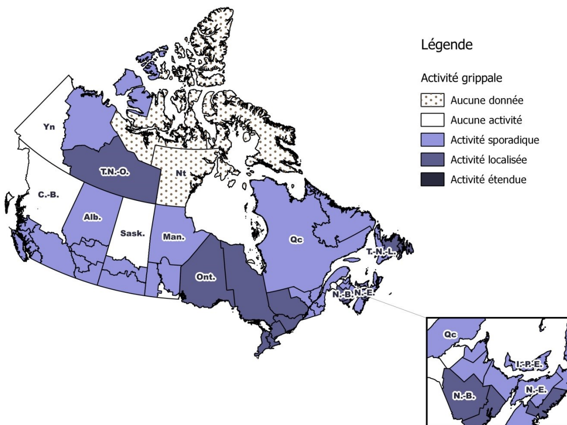
Figure 1 – Carte de l'activité grippale et pseudogrippale globale par province et territoire, Canada, semaine 2018-16
