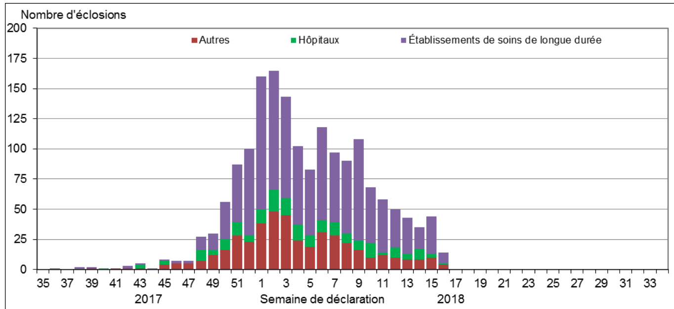
Figure 5 – Nombre total de nouvelles éclosions de la grippe confirmée en laboratoire par semaine, Canada, semaines 2017-35 à 2018-16
