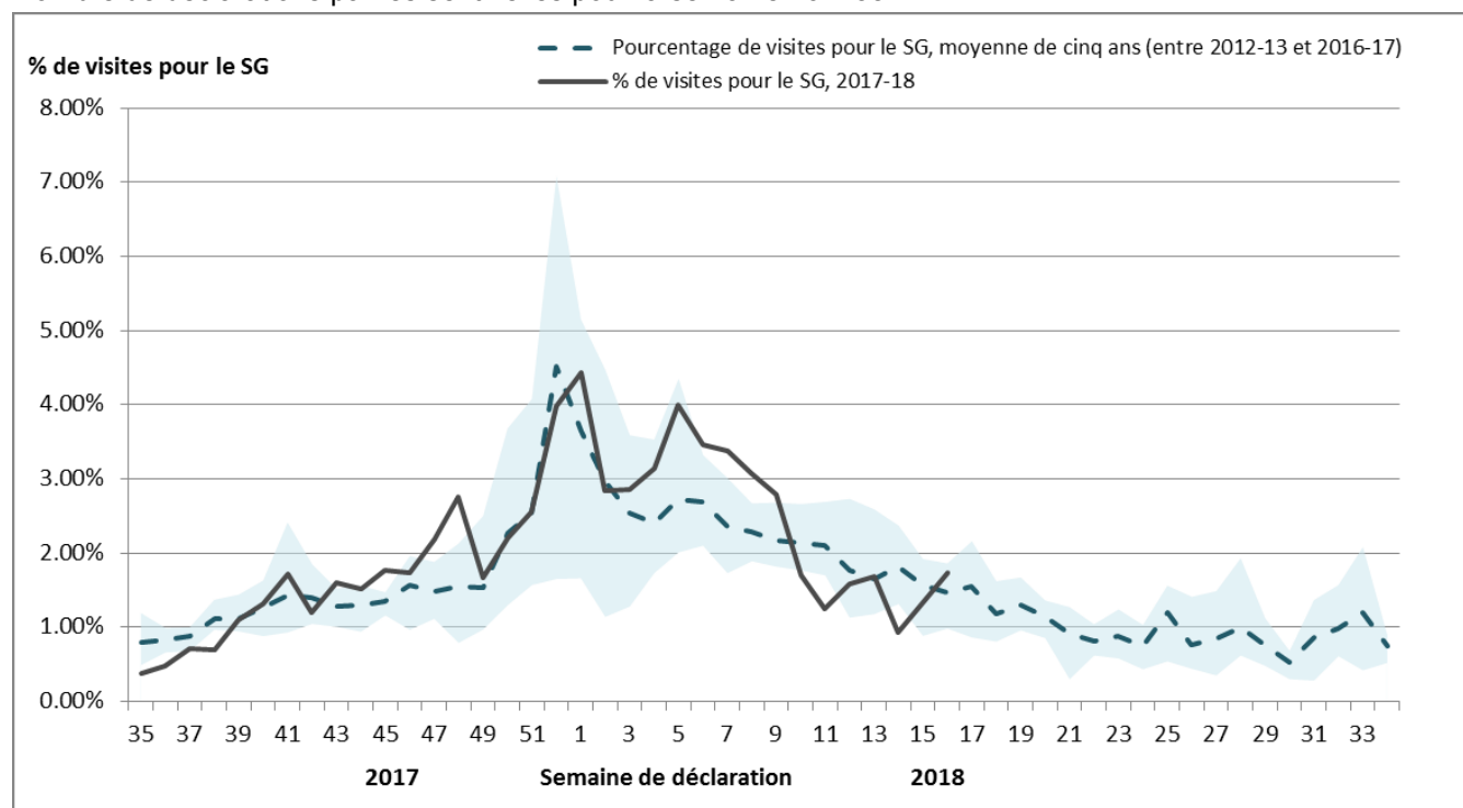
Figure 4 – Pourcentage de visites pour le syndrome grippal déclarées par les sentinelles chaque semaine, Canada, semaines 2017-35 à 2018-16
