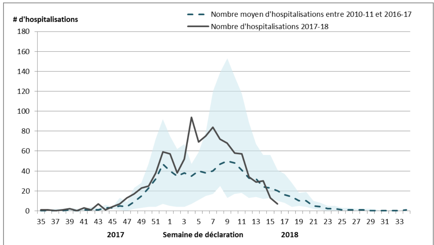
Figure 8 – Nombre d'hospitalisations pédiatriques ( \leq 16 ans) associées à la grippe signalées par le réseau IMPACT, par semaine, Canada, semaines 2017-35 à 2018-16
