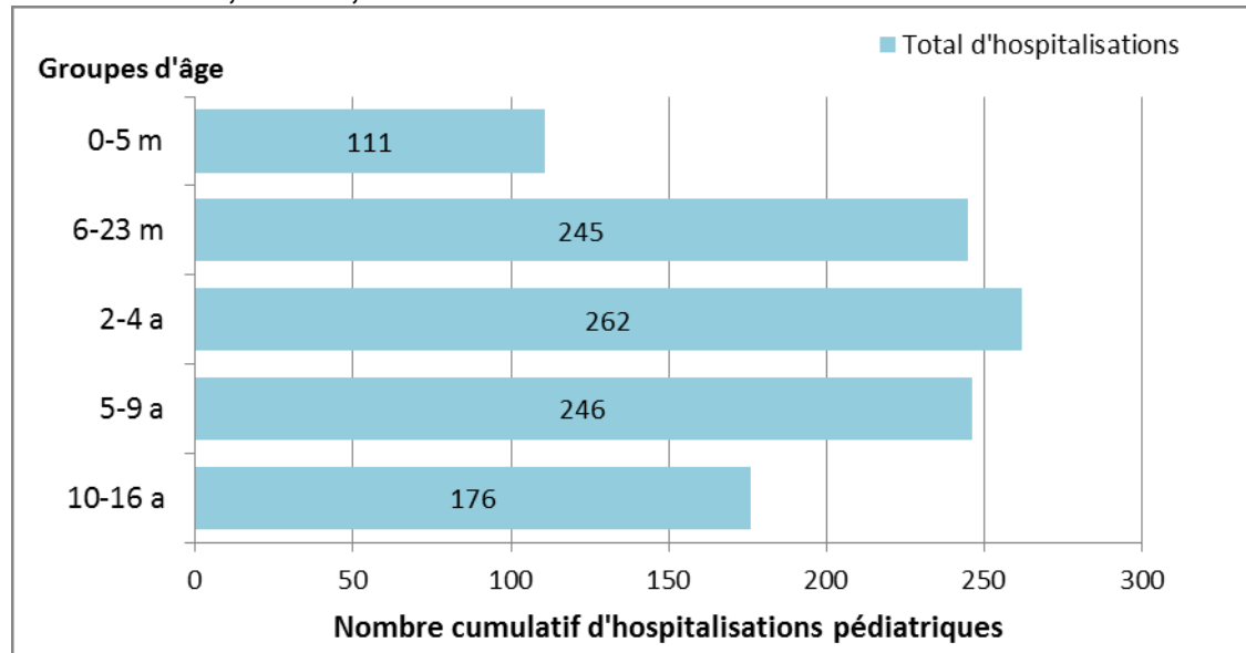
Figure 7 - Nombre cumulatif d'hospitalisations pédiatriques ( \leq 16 ans) associées à la grippe signalées par le réseau IMPACT, Canada, semaines 2017-35 à 2018-16
