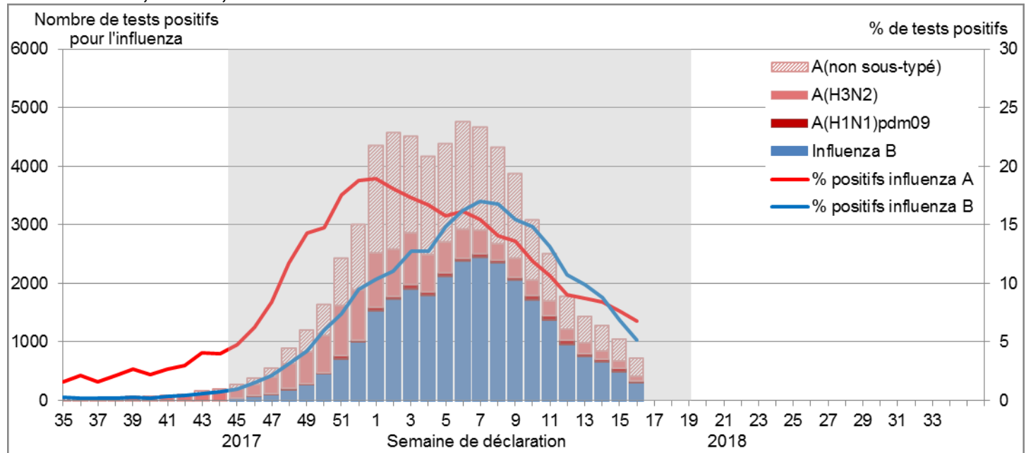
Figure 2 – Nombre et pourcentage de tests de détection de la grippe positifs, par type, sous-type et semaine de surveillance, Canada, semaines 2017-35 à 2018-16
