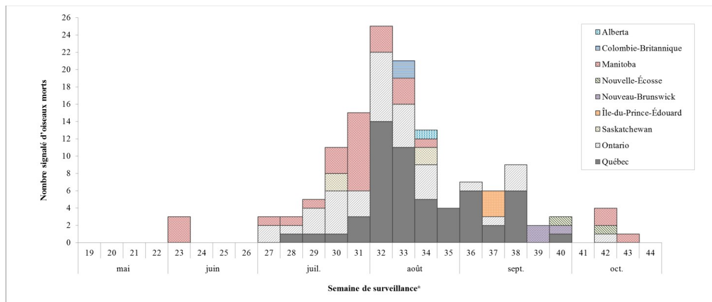
FIGURE 4 : Nombre d'oiseaux sauvages morts positifs au VNO au Canada* par semaine de surveillance ± , 2018
