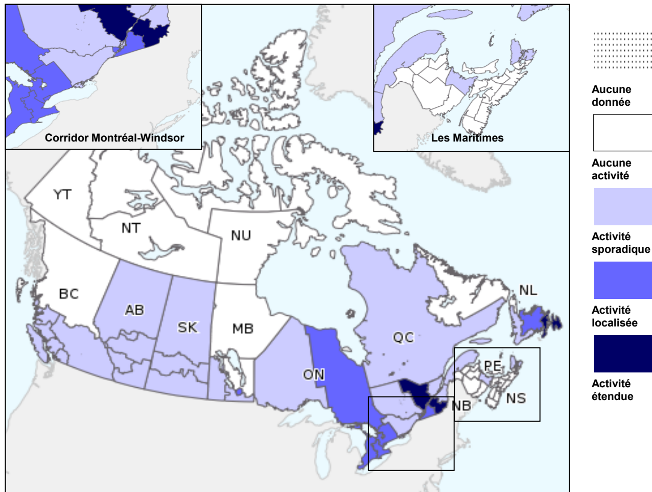
Figure 1. Carte de l'activité grippale et pseudogrippale globale par province et territoire, Canada, semaine 19
