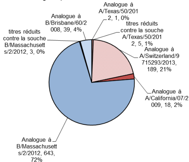
Figure 4. Caractérisation des souches grippales, Canada, 2014-15, N = 898
